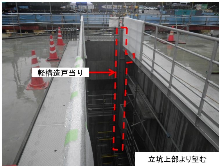
12月4日 軽構造戸当り設置
