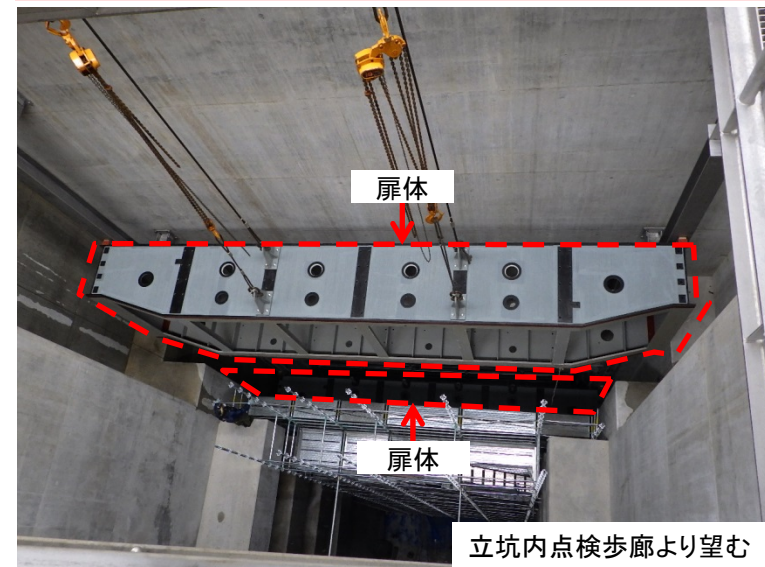
12月25日 扉体組立
