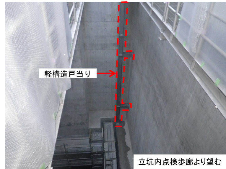
12月11日 軽構造戸当り設置
