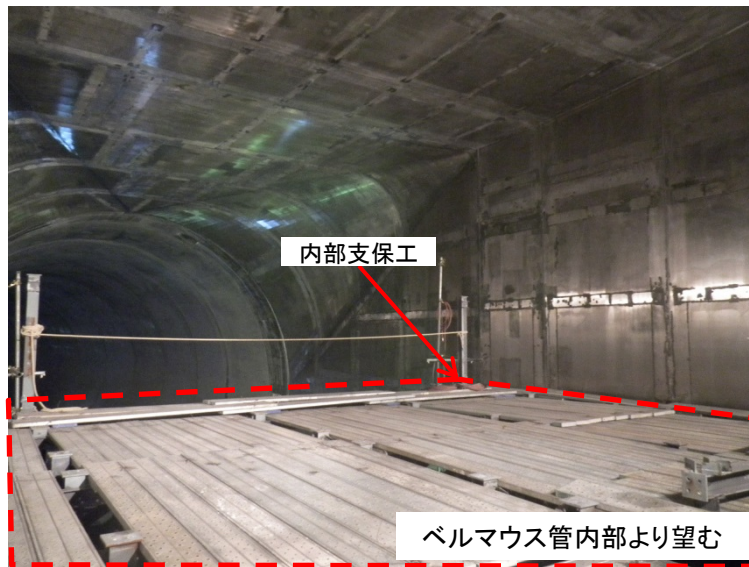
6月5日 ベルマウス管内部支保工(下流部)撤去
