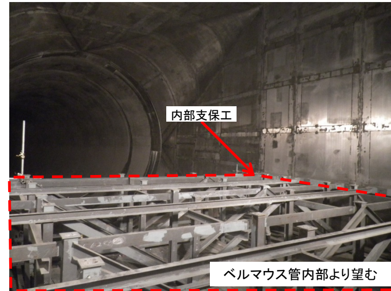
6月12日 ベルマウス管内部支保工(下流部)撤去
