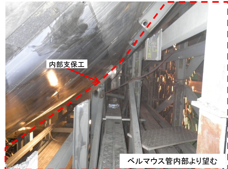
6月26日 ベルマウス管内部支保工(上流部)撤去
