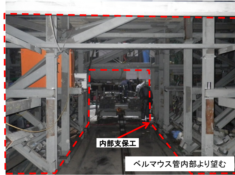
5月15日 ベルマウス管内部支保工撤去
