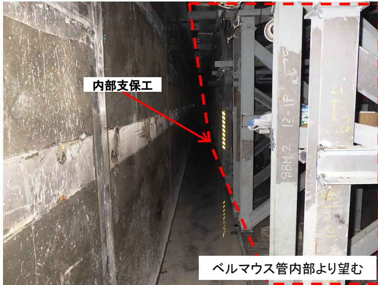
5月8日 ベルマウス管内部支保工撤去
