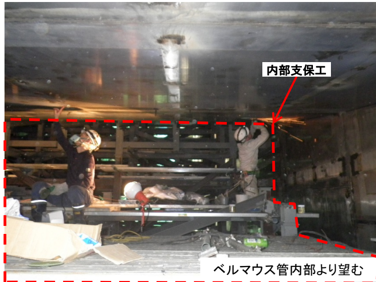
5月22日 ベルマウス管内部支保工撤去
