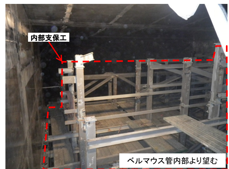
5月29日 ベルマウス管内部支保工撤去
