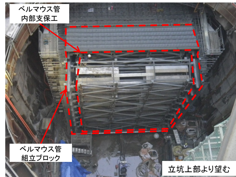
11月14日 ベルマウス管組立
