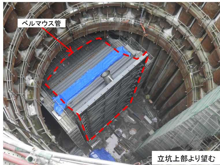
11月21日 ベルマウス管組立完了
