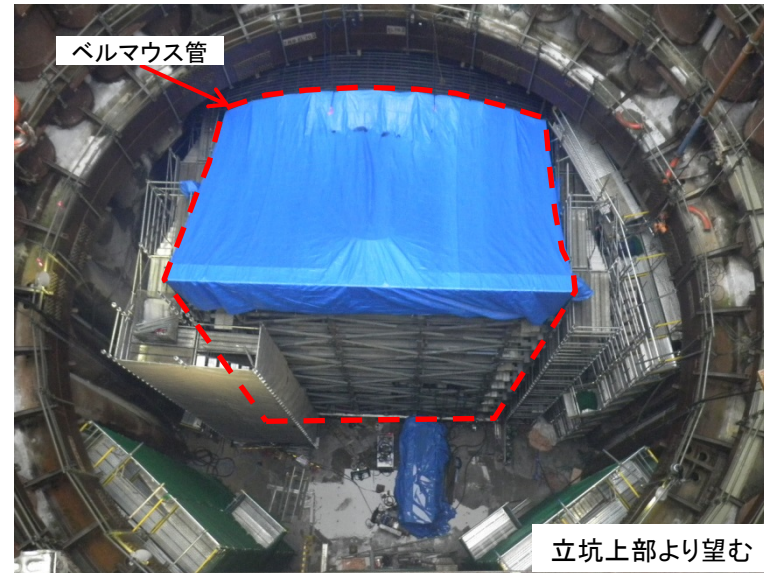
11月28日 ベルマウス管溶接
