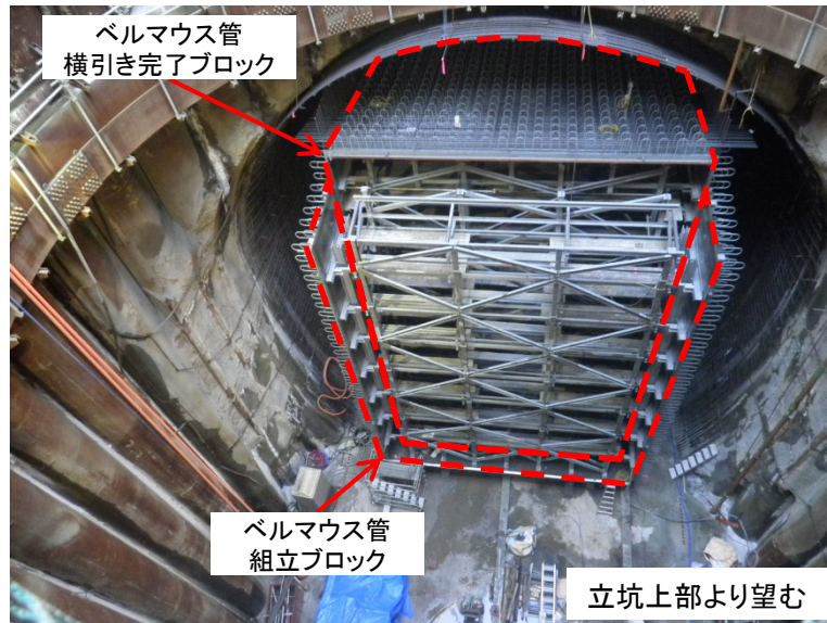
11月7日 ベルマウス管組立
