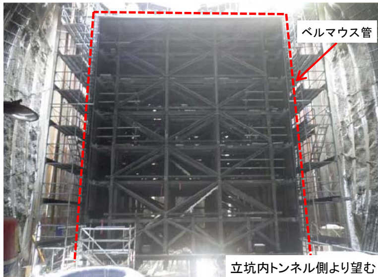
10月17日 ベルマウス管内面ビード盛高調整
