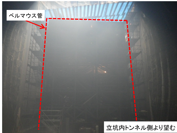
10月3日 ベルマウス管溶接
