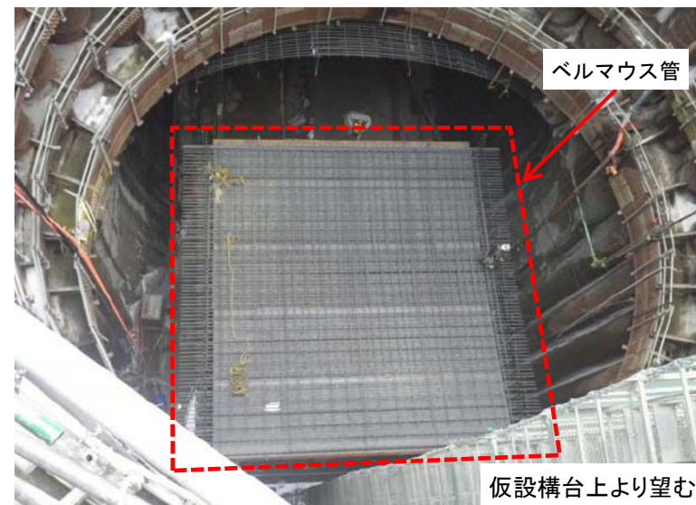
10月24日 ベルマウス管横引き
