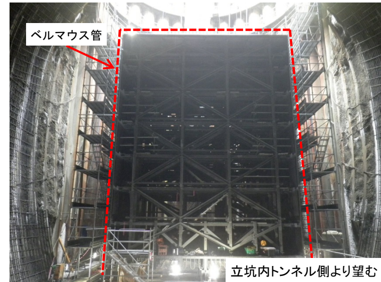
10月10日 ベルマウス管溶接完了
