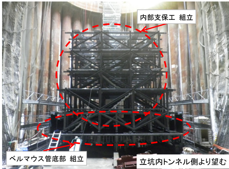
9月5日 ベルマウス管・内部支保工組立
