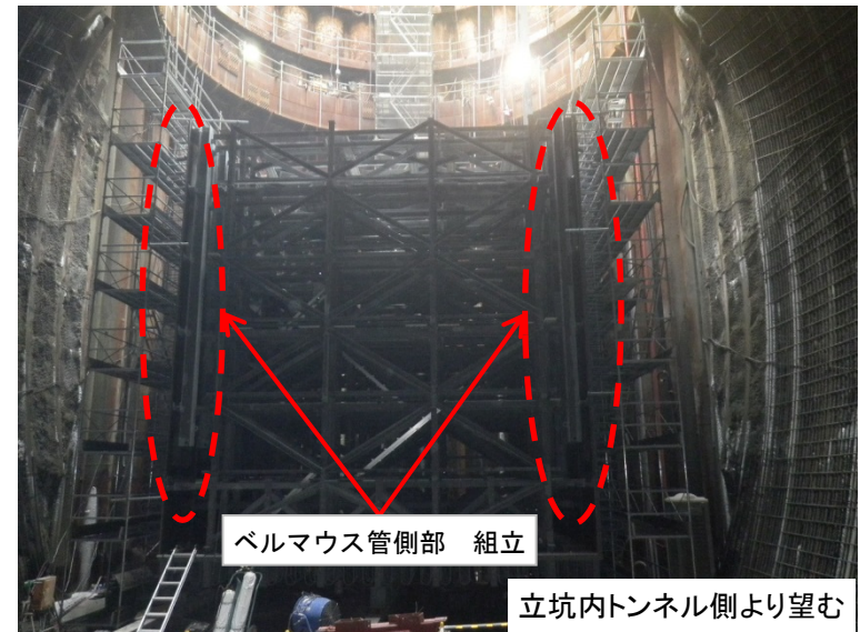
9月12日 ベルマウス管側部組立
