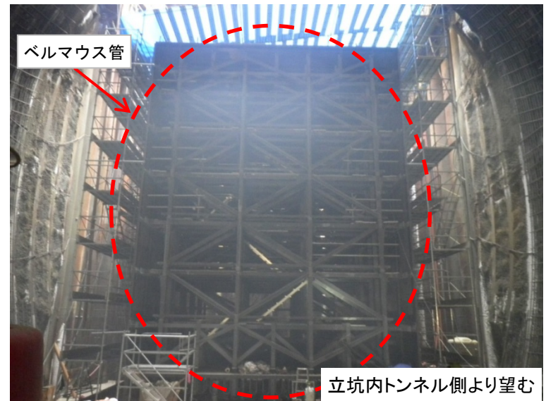
9月26日 ベルマウス管溶接
