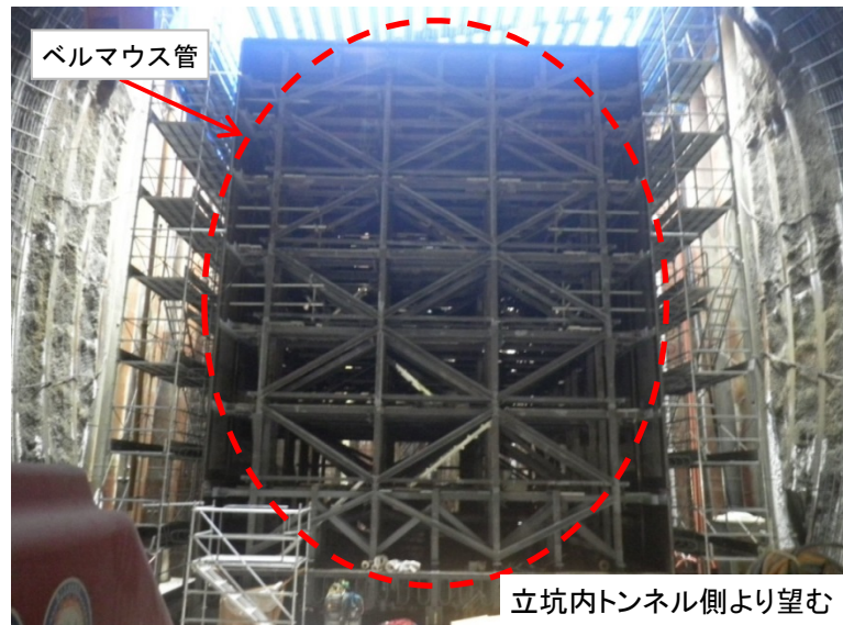
9月19日 ベルマウス管組立完了
