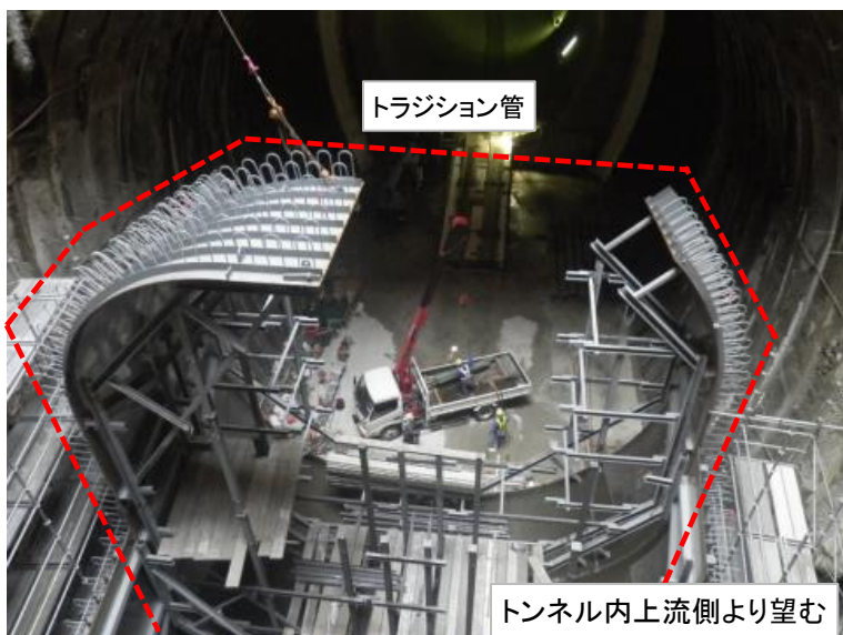
4月18日 トランジション管組立
