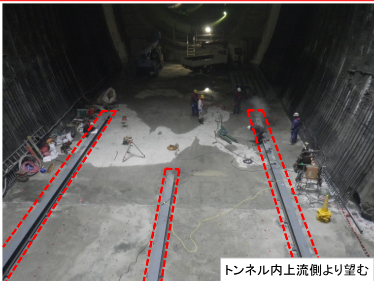
4月4日 引込レール据付
