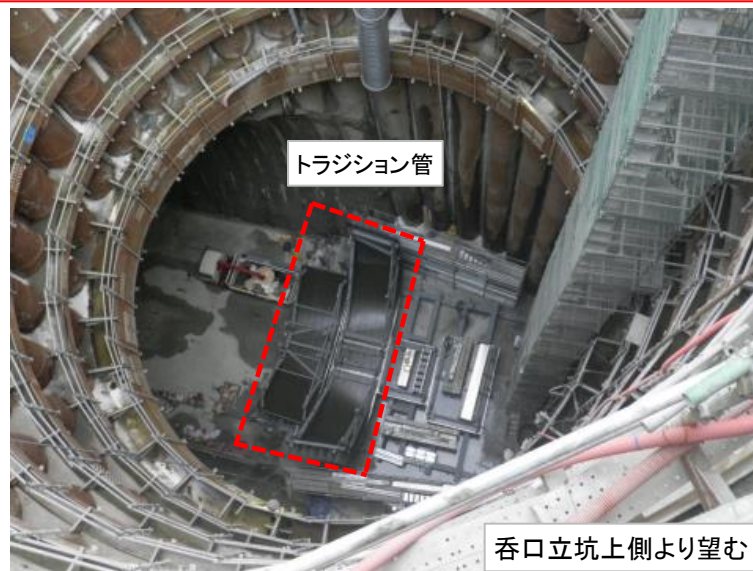
4月11日 トランジション管組立
