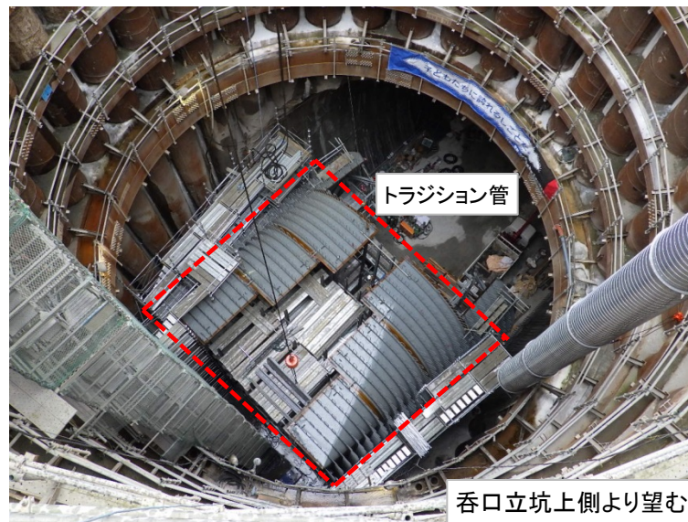
4月25日 トランジション管組立
