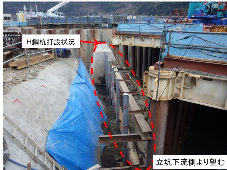
1月10日 軽量盛土壁面H鋼杭打設状況
