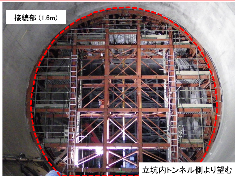
11月7日 覆エコンクリート養生中
