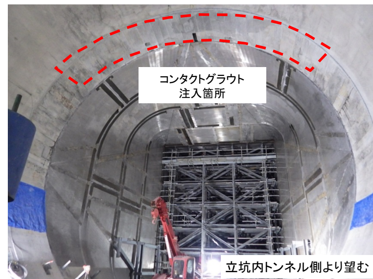
11月28日 コンタクトグラウト注入準備
