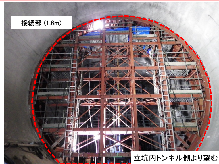
11月14日 バラセトル(組立式型枠)の撤去準備
