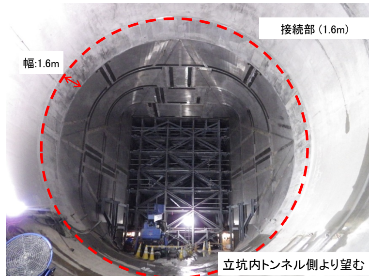
11月21日 バラセトル(組立式型枠)の撤去完了
