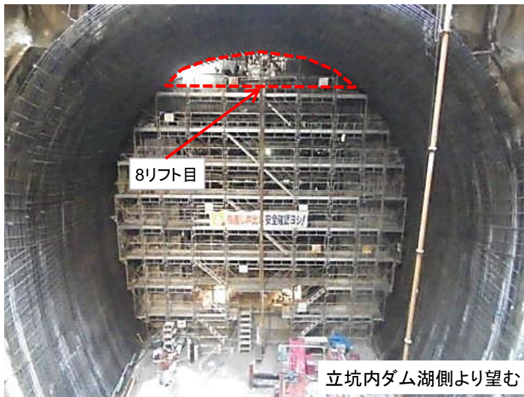
8月1日 コンクリート打設(8リフト目)
