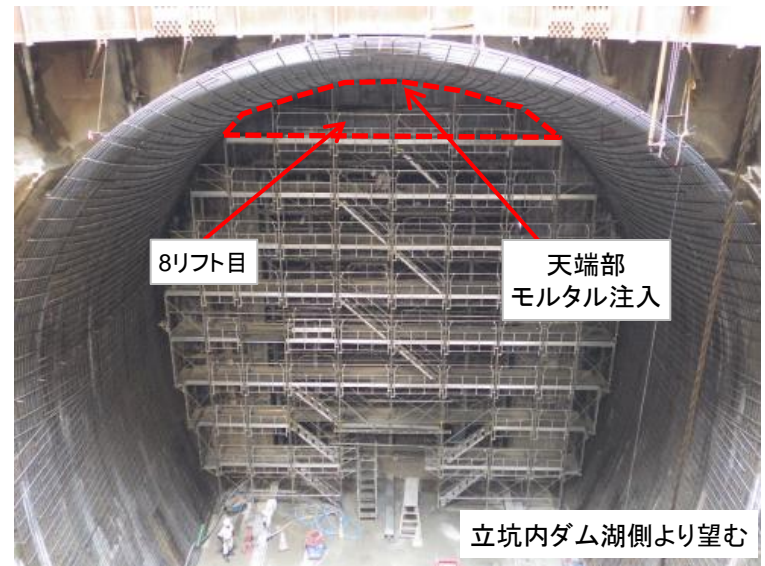
8月8日 天端部モルタル注入完了
