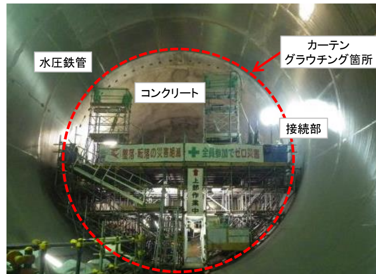
4月11日 カーテングラウチング
