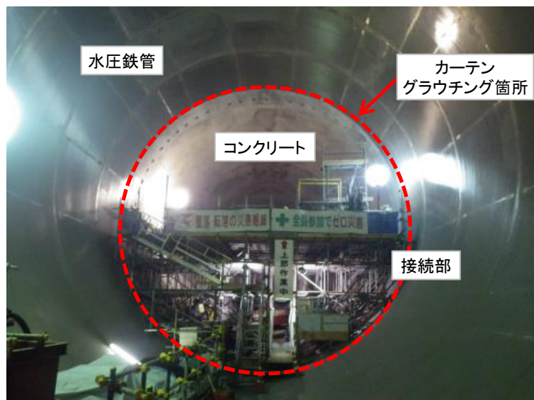
4月18日 カーテングラウチング
