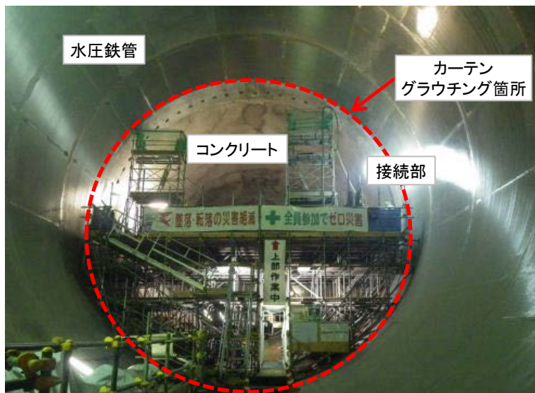
4月4日 カーテングラウチング
