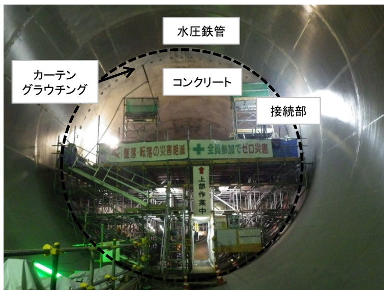
3月7日 カーテングラウチング
