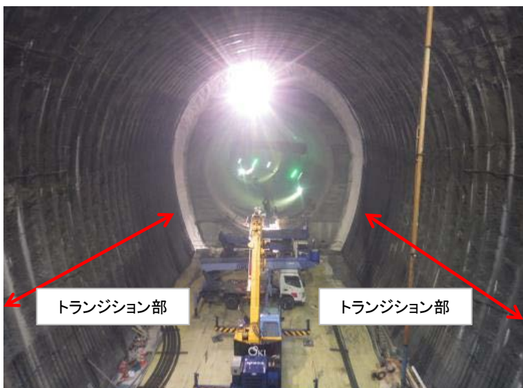
3月22日 外周鉄筋組立(トランジション部)
