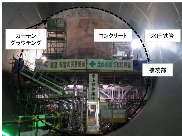
3月22日 カーテングラウチング
