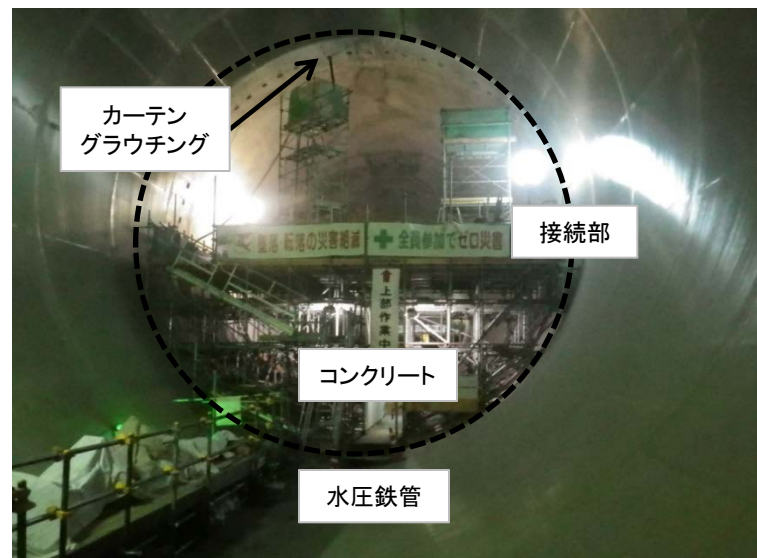
3月14日 カーテングラウチング
