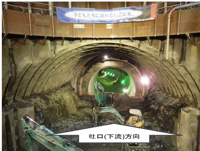
12月21日 立坑内迎え掘り掘削
