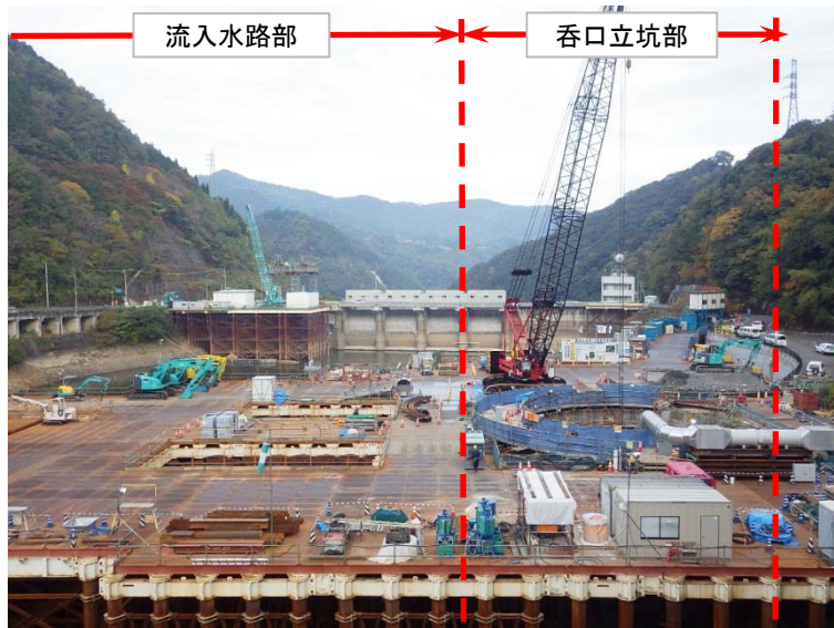
11月2日 立坑内迎え掘り掘削
