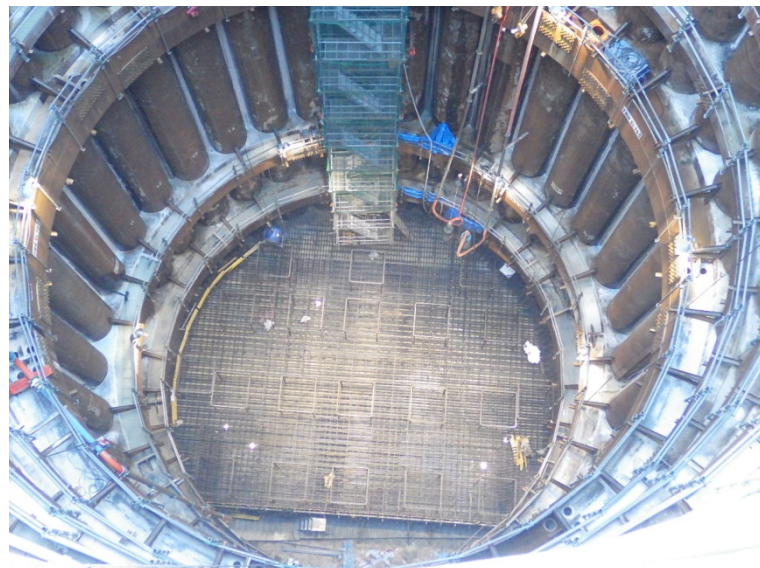
9月7日 立坑掘削、鋼管背面ミルク注入削孔
