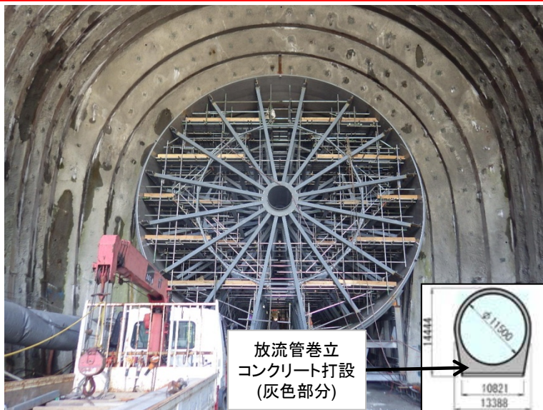
6月1日 放流管巻立コンクリート打設、レール撤去
