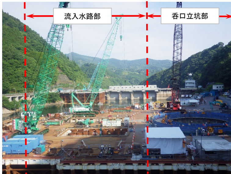
6月1日 鋼管矢板建込、立坑掘削、鋼管内カーテングラウト
