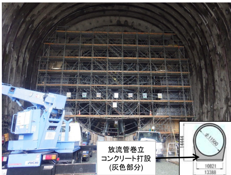
6月15日 放流管巻立コンクリート打設、内部支保工解体
