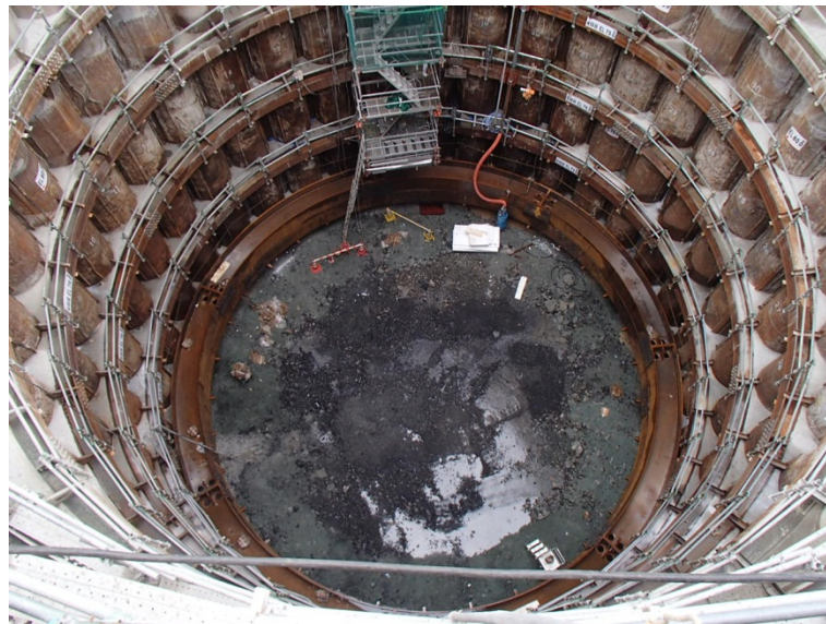
6月15日 鋼管矢板建込、立坑掘削、鋼管内カーテングラウト
