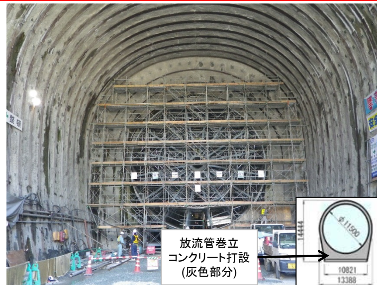
6月8日 内部支保工解体
