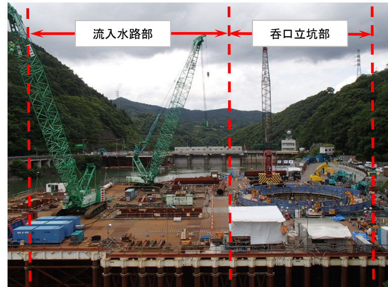
6月22日 鋼管矢板建込、立坑掘削、鋼管内カーテングラウト
