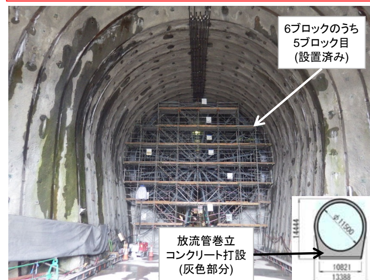
5月25日 放流管巻立コンクリート打設、内部支保工解体
