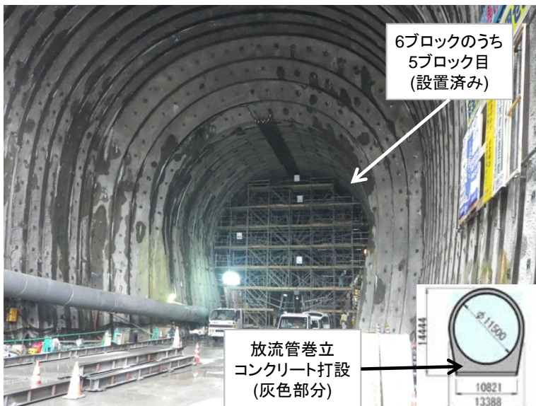
5月18日 放流管巻立コンクリート打設、内部支保工解体
