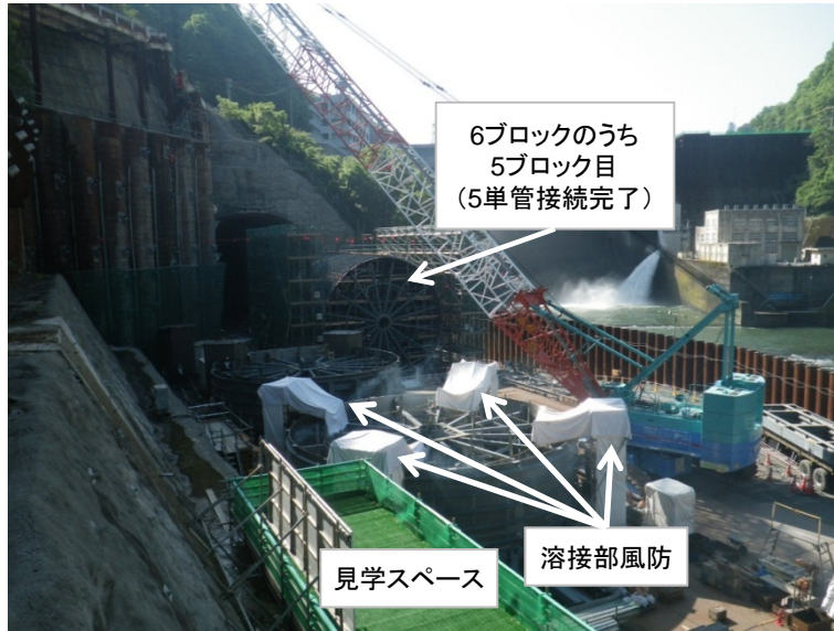
5月4日 放流管組立、放流管トンネル坑内搬入
