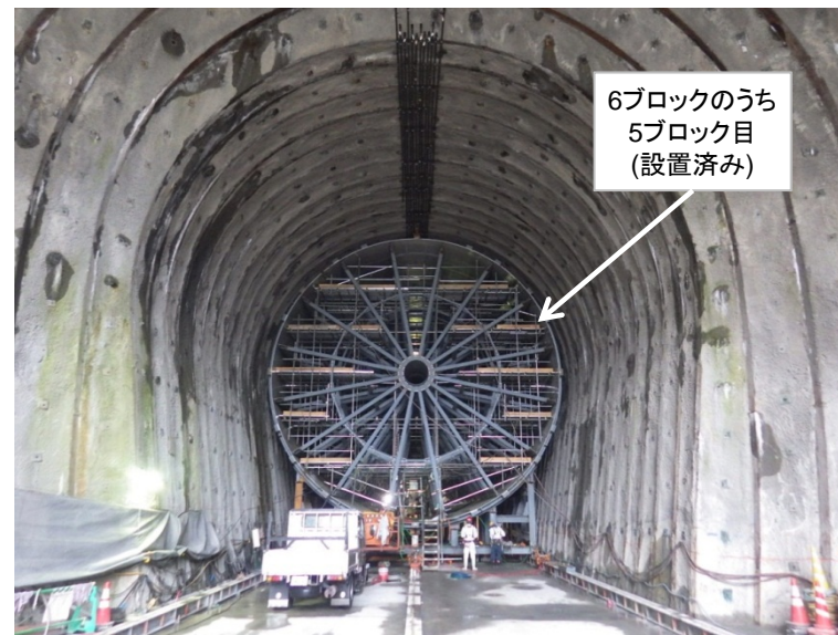
5月11日 放流管巻立コンクリート打設、放流管連結、内部支保工解体
