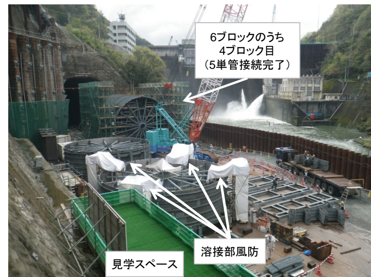
4月13日 放流管組立
