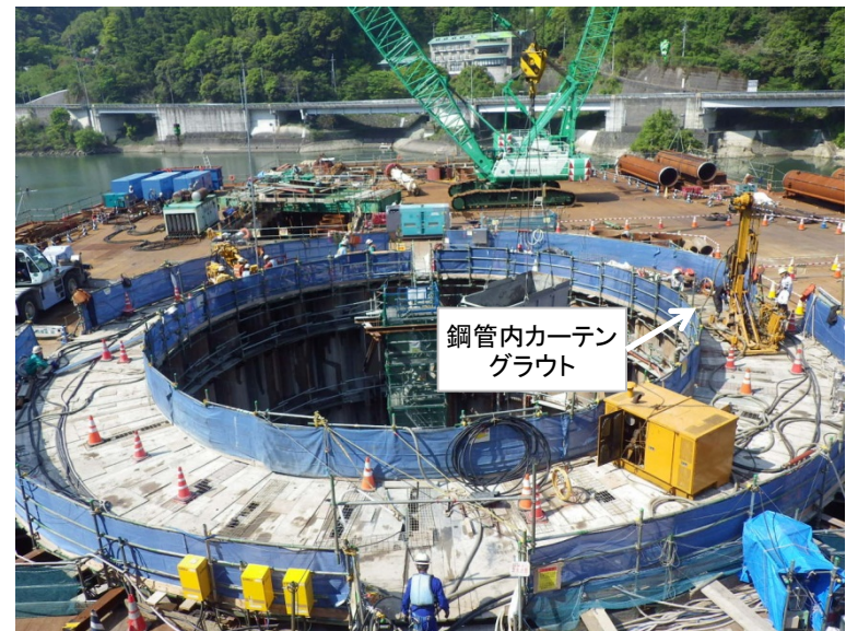
4月27日 鋼管矢板建込、鋼管内カーテングラウト、立坑掘削
