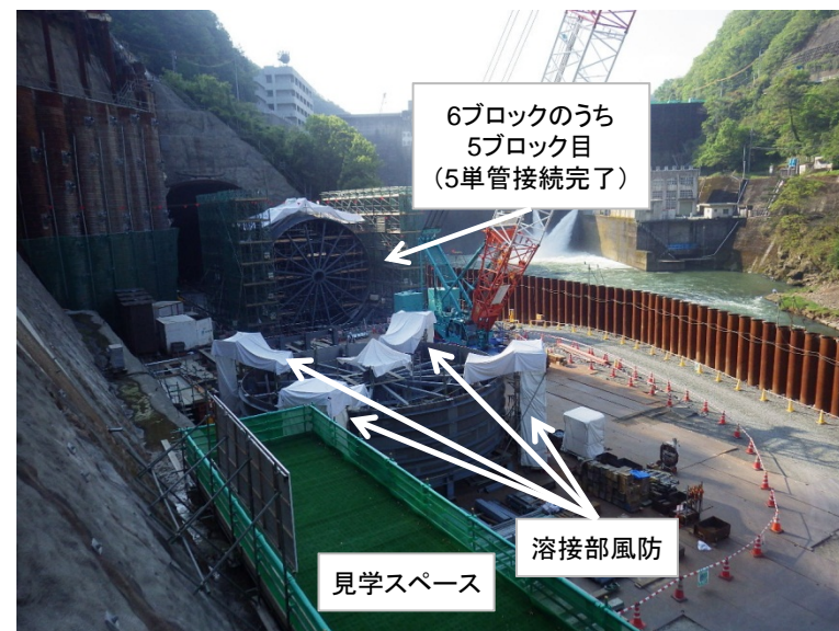
4月27日 放流管組立
