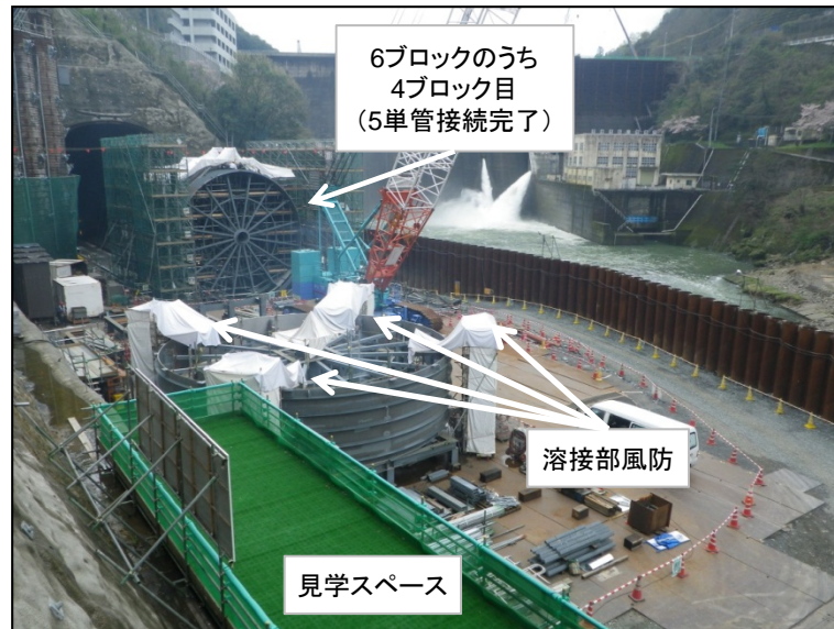
4月6日 放流管組立、放流管トンネル坑内搬入
