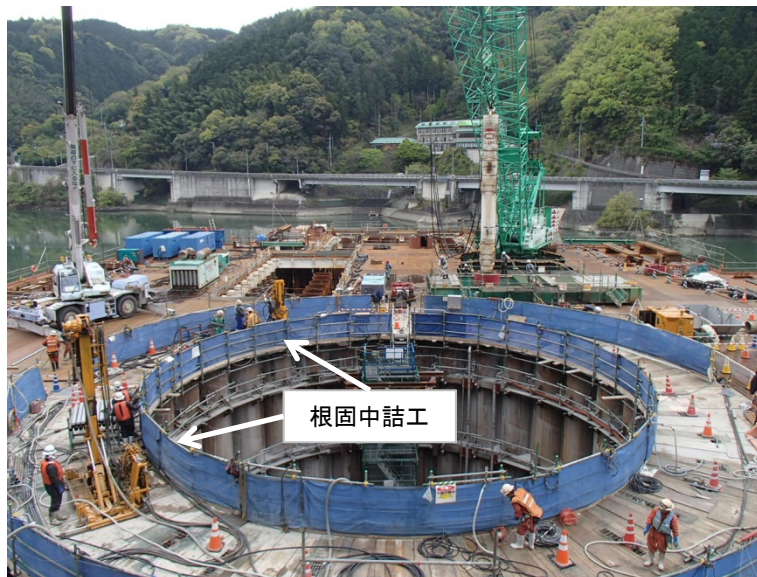
4月20日 鋼管矢板建込、根固中詰工、立坑掘削
