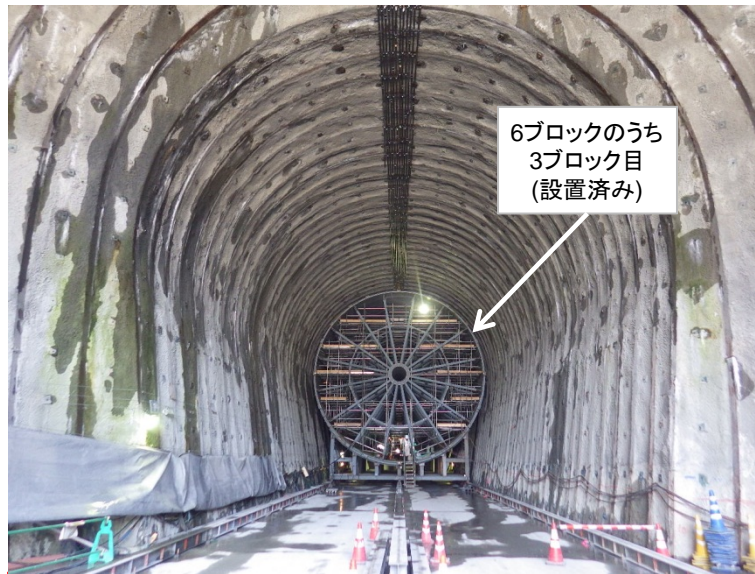
4月20日 放流管巻立コンクリート打設
