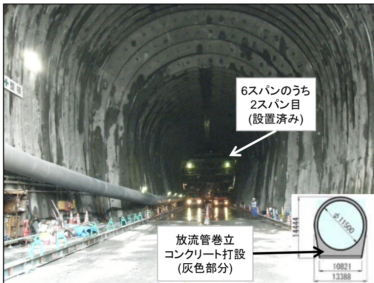
3月16日 放流管巻立コンクリート打設、放流管連結
