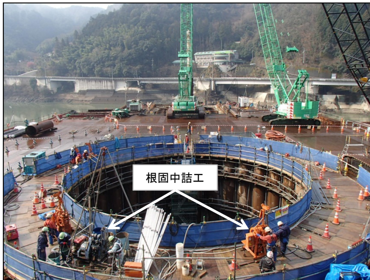
3月16日 鋼管矢板建込、根固中詰工、立坑掘削
