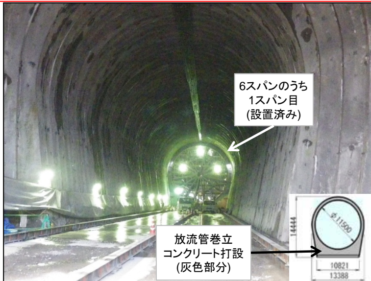
3月2日 放流管巻立コンクリート打設
