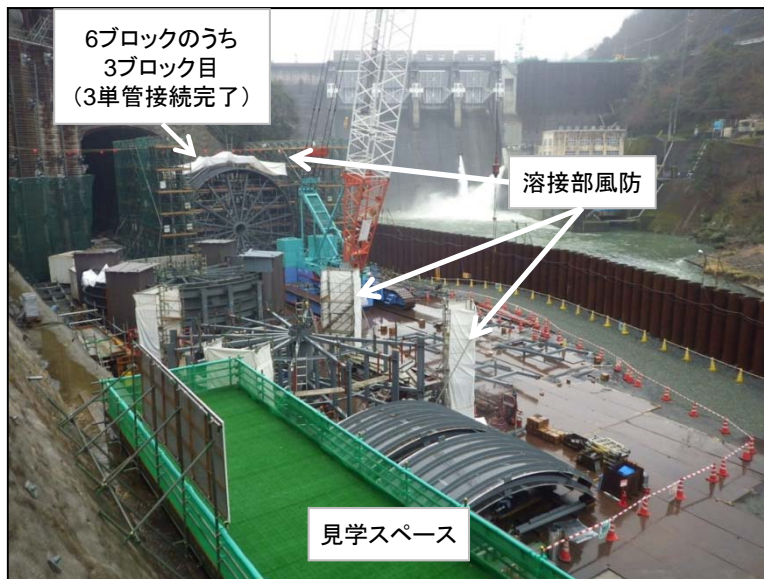
3月16日 放流管組立
