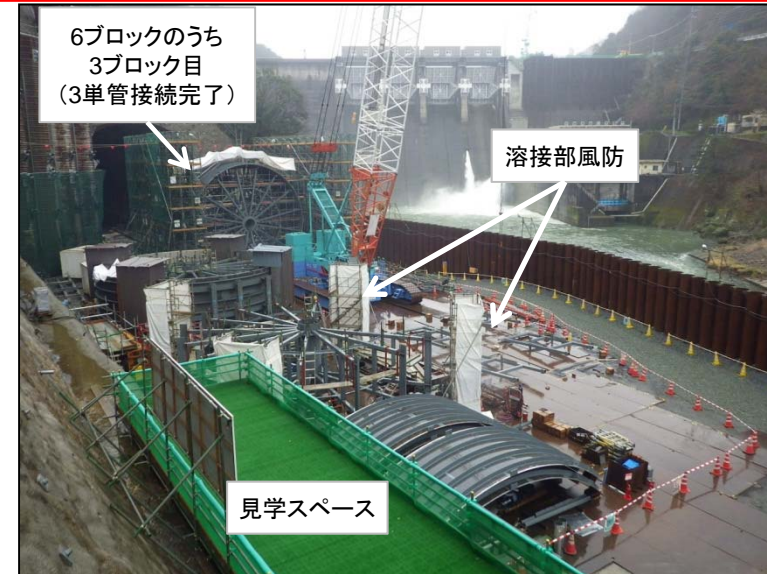
3月9日 放流管組立
