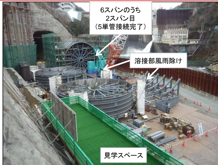
3月2日 放流管組立、放流管トンネル坑内搬入
