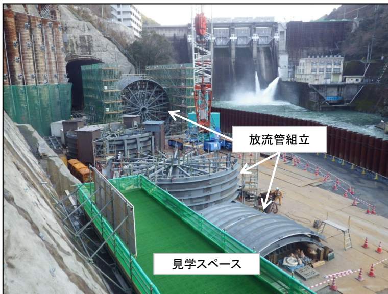
1月19日 放流管組立
