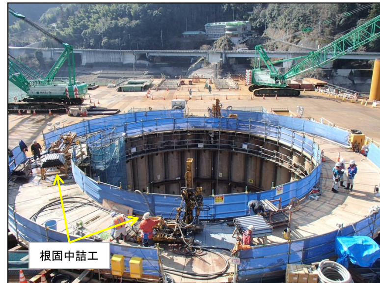
1月26日 鋼管矢板建込導枠設置、根固中詰工
