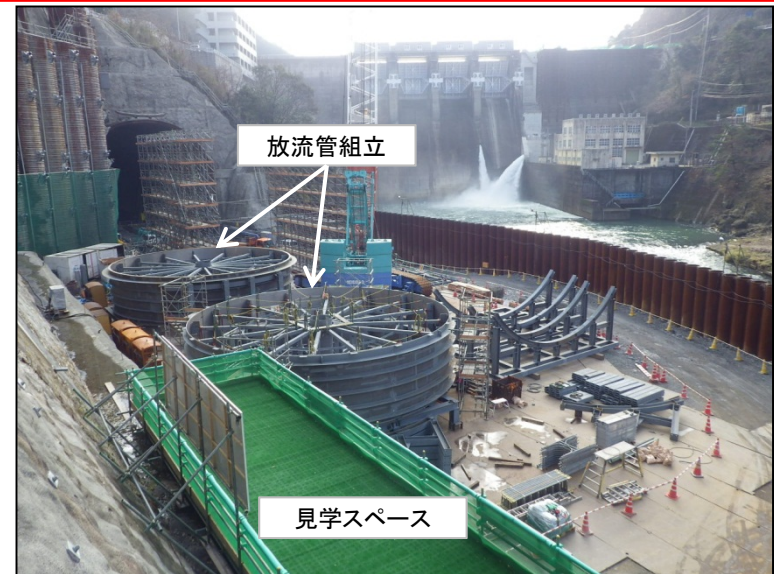
1月13日 放流管組立
