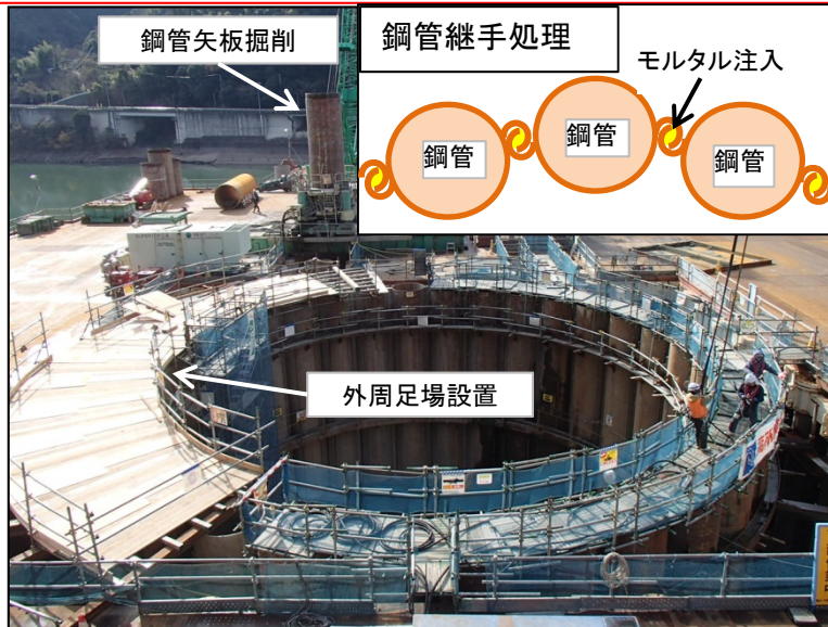
1月5日 鋼管矢板部掘削、鋼管継手処理工
