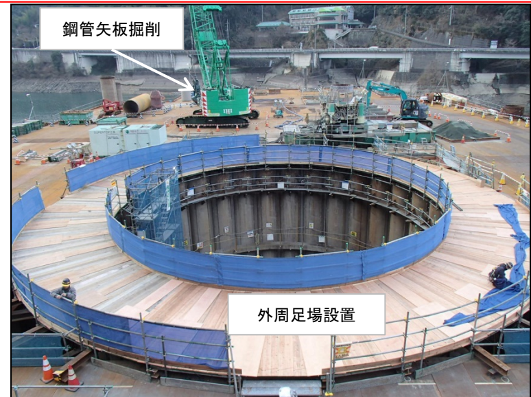
1月13日 鋼管矢板部掘削、鋼管継手処理工
