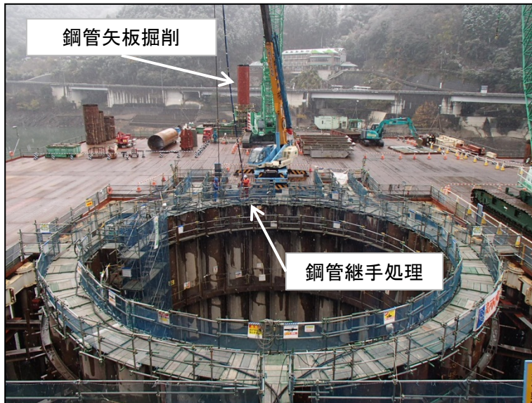
12月15日 鋼管矢板部掘削、鋼管継手処理工
