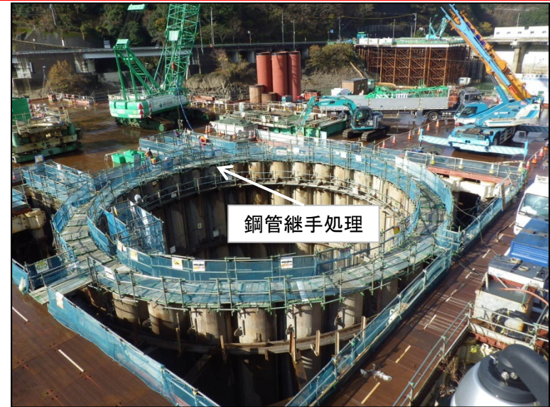
12月8日 鋼管矢板部掘削、鋼管継手処理工
