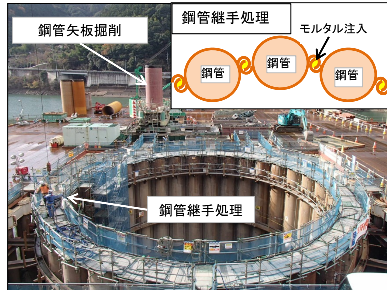
12月22日 鋼管矢板部掘削、鋼管継手処理工
