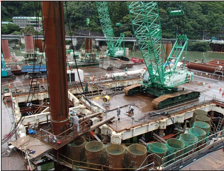
8月4日 流入水路掘削、鋼管矢板打込み
