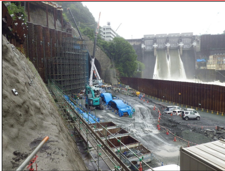
8月4日 深礎アンカー工足場組立、深礎アンカー工
