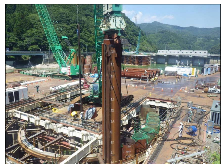
7月28日 流入水路掘削、鋼管矢板打込み
