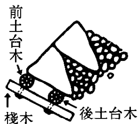
図3 梯子土台
