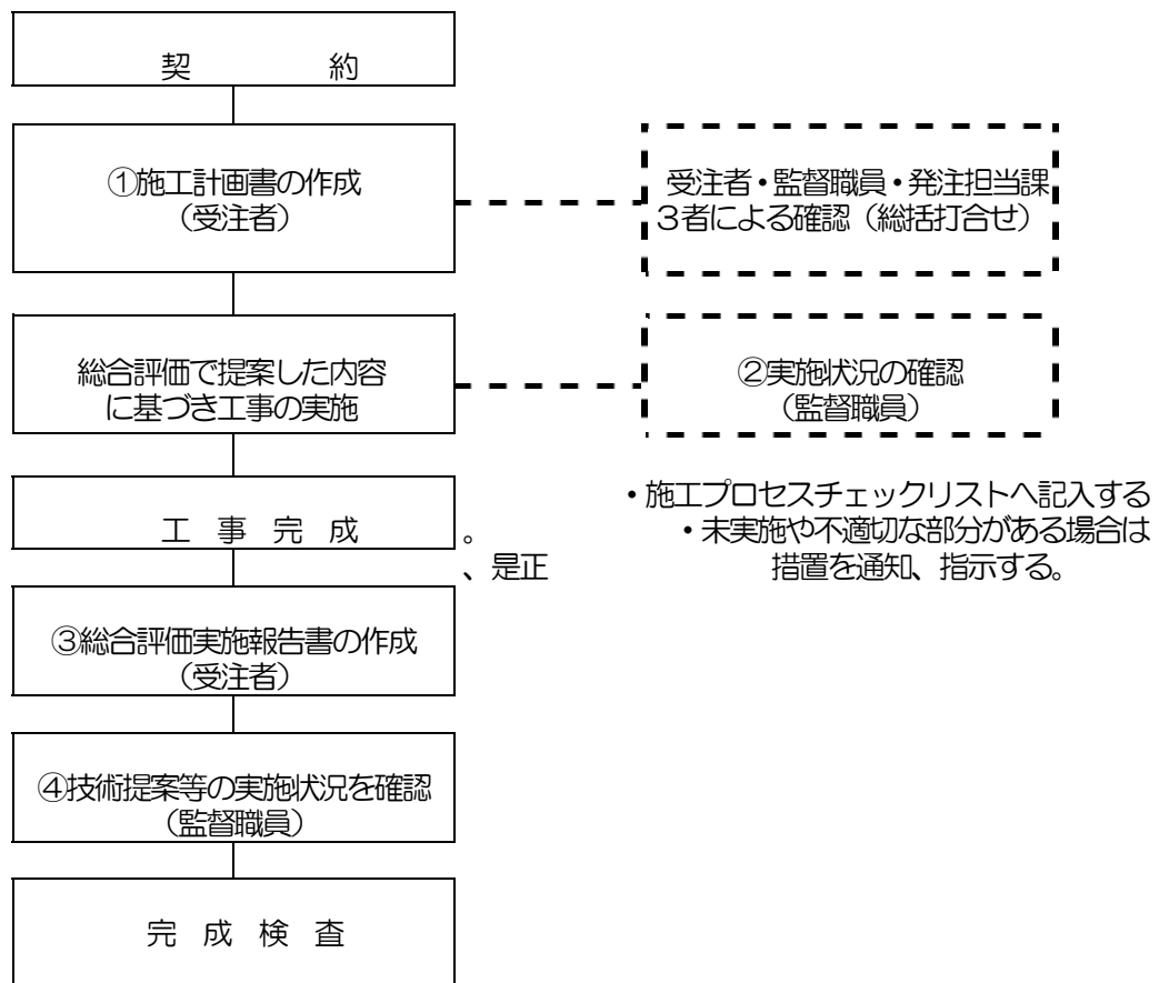
技術提案の確認フロー
